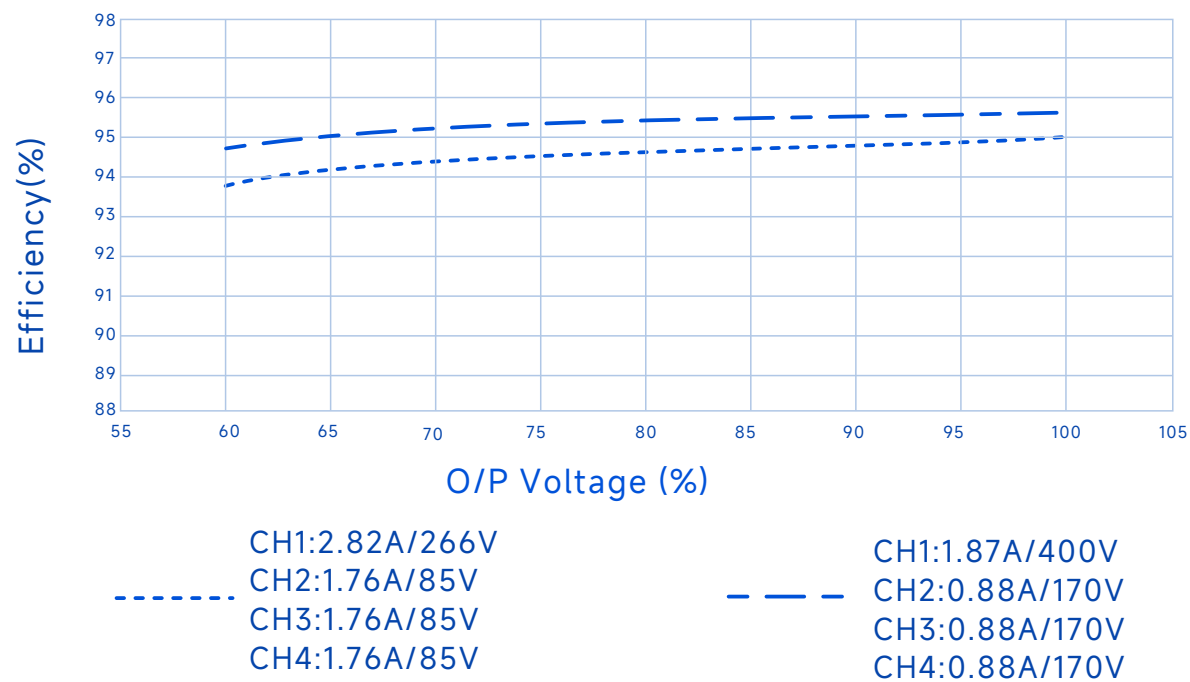
效率Vs.输出电压(Vin=400Vac)
